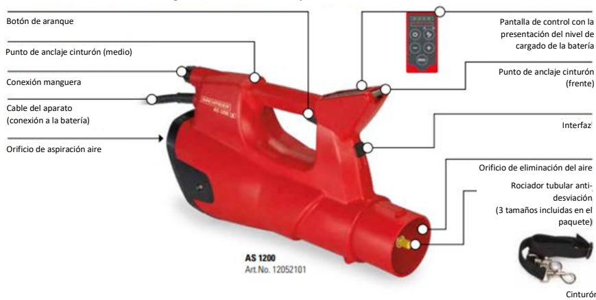
Pulverizador AS 1200 con batería, cargador e unidad de transporte de la batería
